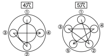
「ナットの締め付け順序」
